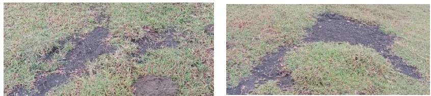
Gambar 3.3 geologi
