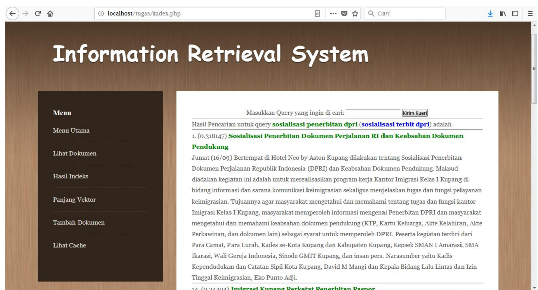
Gambar 4.1 Hasil pencarian terhadap query “sosialisasi penerbitan dpri”
