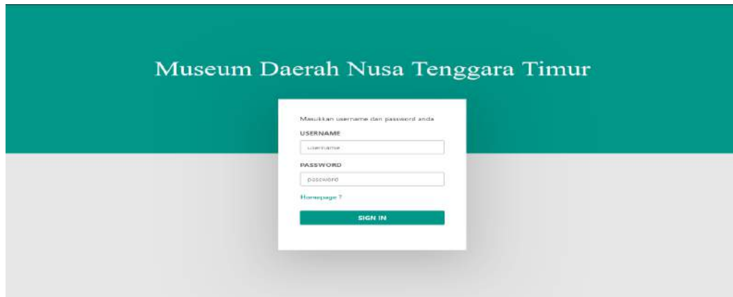
Gambar 4.13 Halaman Login
